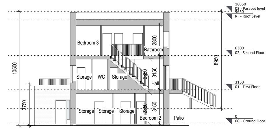
③ Section 1 1 : 200
